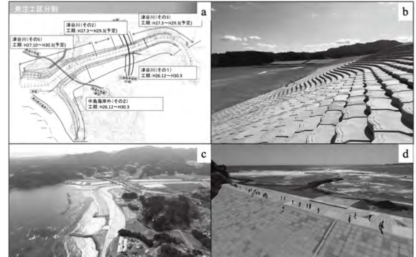
図 2 小泉地区中島海岸の防潮堤の計画と完成した様子 (a) 設計段階、完成した後の (b) 海側の法面の様子、(c)(d) 上空から見た様子。(a)(c)(d) は、中島海岸及び津谷川災害復旧工事を担った五洋・みらい・徳倉特定建設工事共同企業体ホームページより引用 [20]。(b) は 2019 年 10 月 9 日筆者が撮影。
